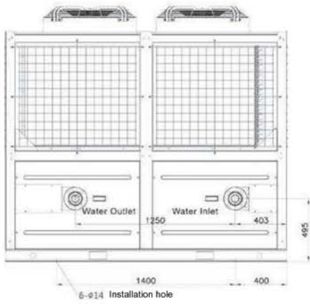
30RAM201XC 30RHM201XH
