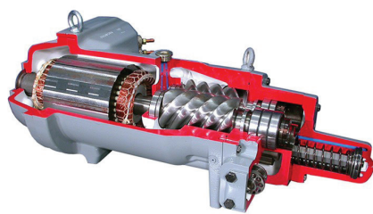
Compressori
